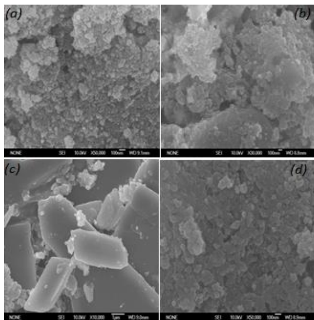
Fig. 1. SEM images of LDHs (a) Mg-Al(OH)_2PO_4 , 1 (b) Mg-Al(OH)_2PO_4PF_6 , 2 (c) Ca-Al(OH)_2SO_4 , 3 and (d) Ca-Al(OH)_2PO_4PF_6 , 4. (Khansi et al., 2018)
